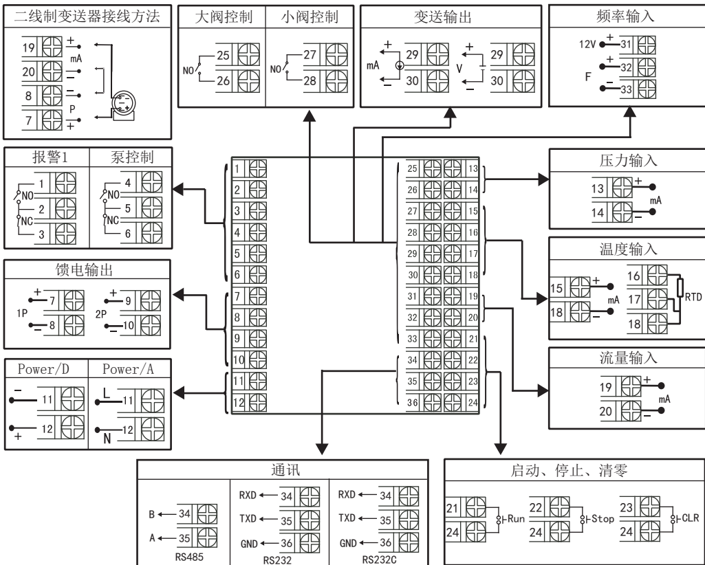
OHR-F672接线图
