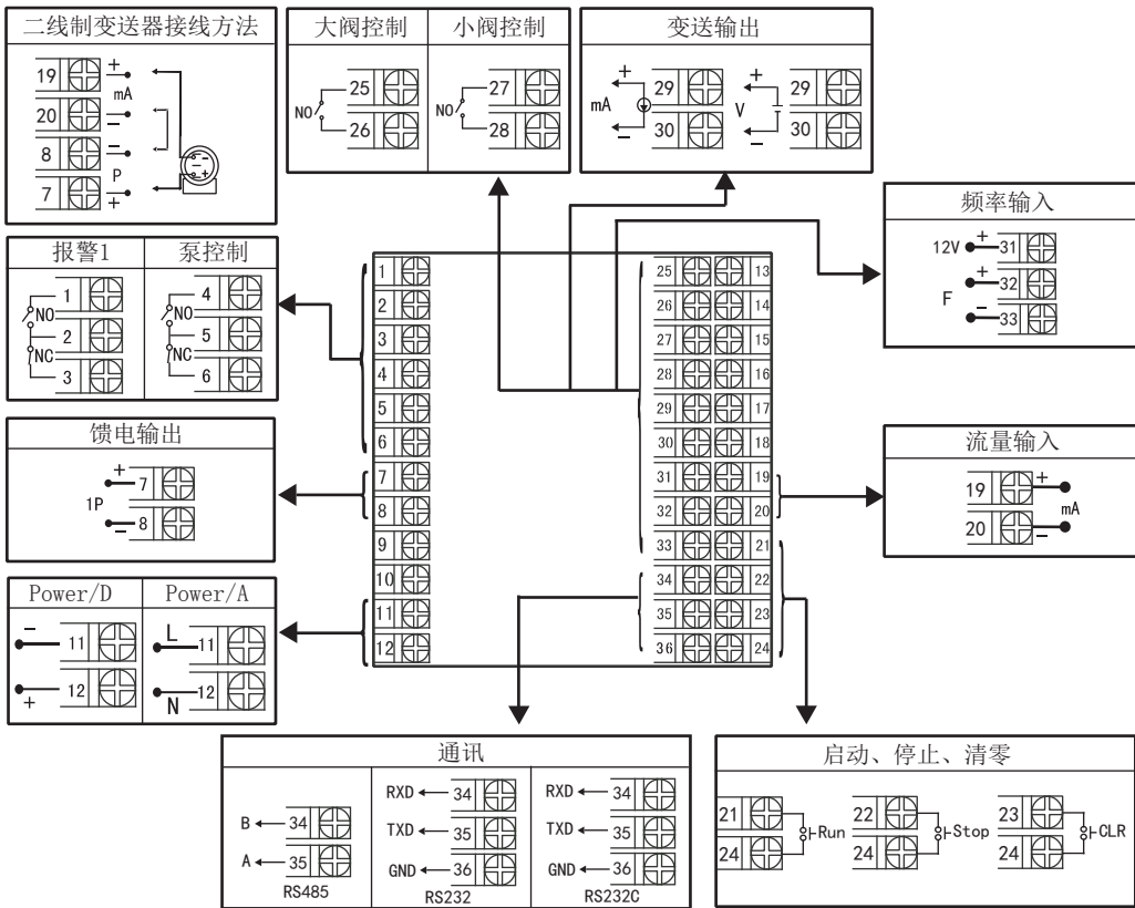
OHR-F671接线图
